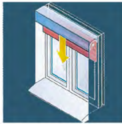
Pose traditionnelle (coffre titan)
